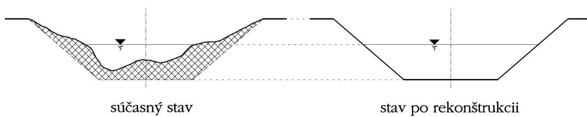
Obr. X.4. Schéma rekonštrukcie kanála
