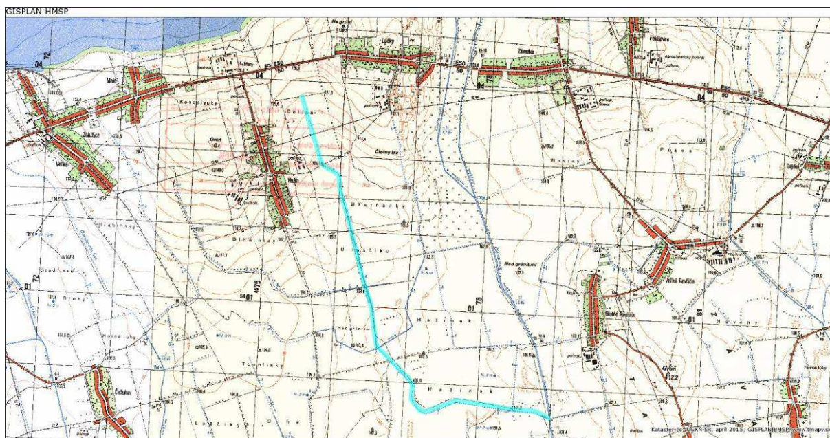
Obr. X.1. Prehľadná situácia kanála Hažínsky (ev. č. 5 405 042 004) na území obce Hažín
