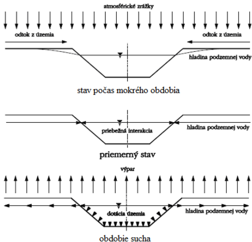
Obr. X.6. Schéma funkcie kanála počas vodného obdobia, priemerného stavu a obdobia sucha (priečny profil)
